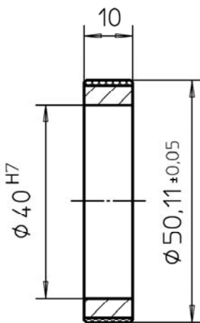
50770-KR108 Innendurchmesser variabel
