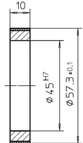
50835-KR121 Innendurchmesser variabel
