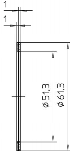
50723-KR97 Innendurchmesser fix
