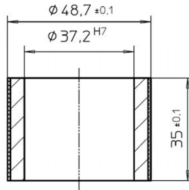
50832-KR118 Innendurchmesser variabel
