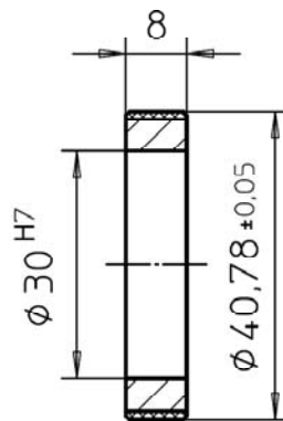
50836-KR122 Innendurchmesser variabel
