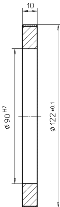
50802-KR117 Innendurchmesser variabel
