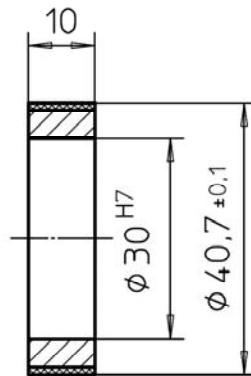
50834-KR120 Innendurchmesser variabel
