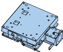
Encoder
